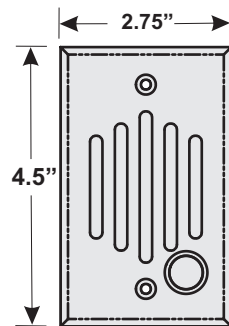
IU-Series Intercom
